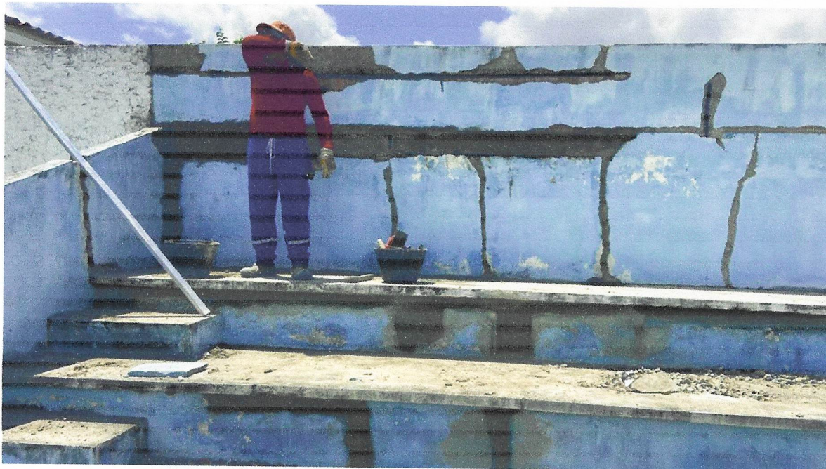
Foto 03- ALVENARIA DE VEDAÇÃO DE BLOCOS CERÂMICOS FURADOS NA VERTICAL DE 9X19X39 CM (ESPESSURA 9 CM) E ARGAMASSA DE ASSENTAMENTO COM PREPARO MANUAL. AF_12/2021
